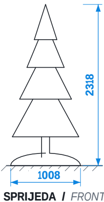
SPRIJEDA / FRONT
