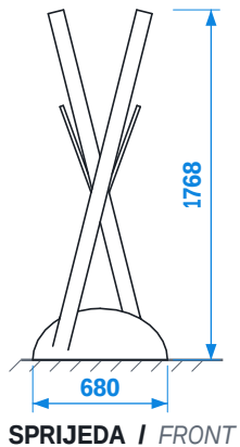
SPRIJEDA / FRONT
